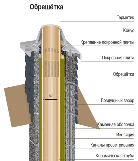
Выполняемая по месту обрешётка
