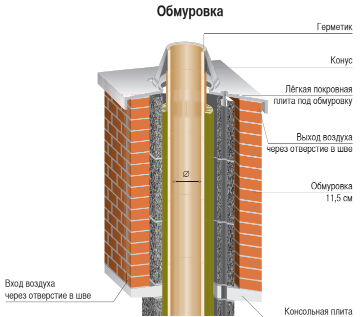
Выполняемая по месту обмуровка на консольной плите
