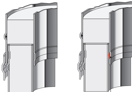
Уплотнительная манжета для работы с конденсационными котлами или при избыточном давлении до 200 Па. Ограничение по температура газов: до 200 гр. С
