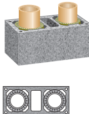
Двухходовой дымоход с вентиляционным/многофункциональным каналом
